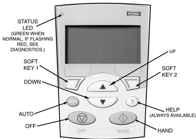
Fig. 131 — VFD Keypad (P/N ACH-CP-H)
